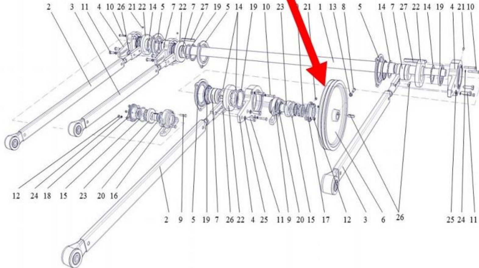
Рис. 10 СВУ60.05.000А
